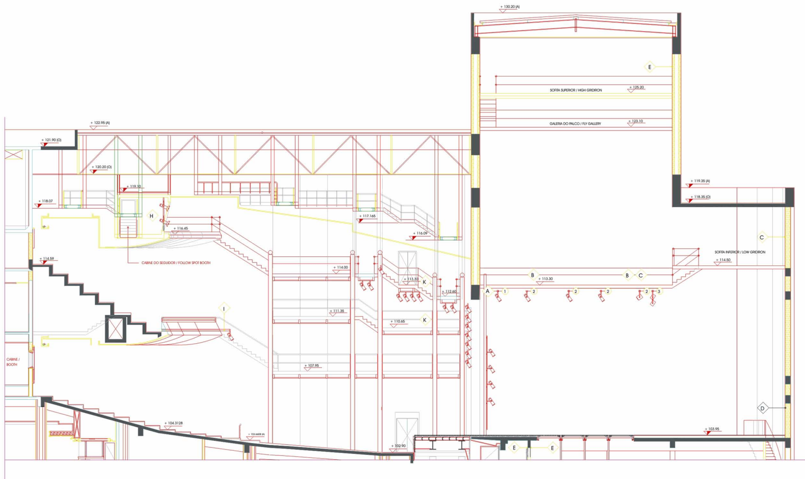
CORTE AA ILUMINAÇÃO / LIGHTING SECTION AA
