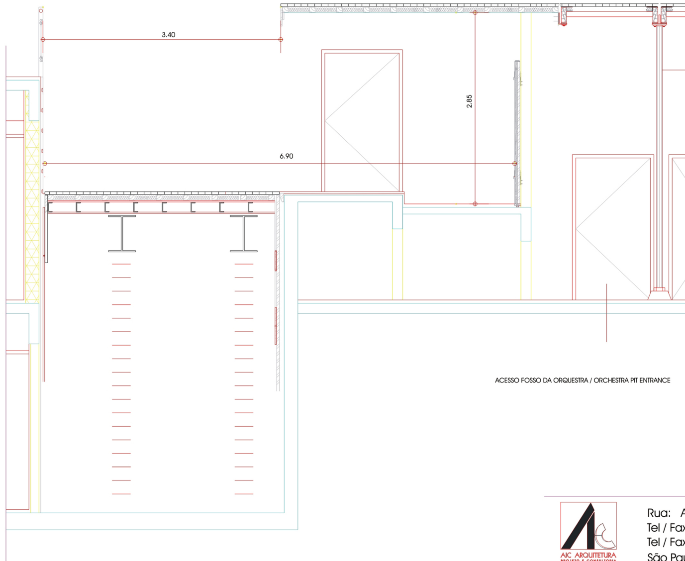
DETALHE FOSSO DA ORQUESTRA / ORCHESTRA PIT DETAIL
